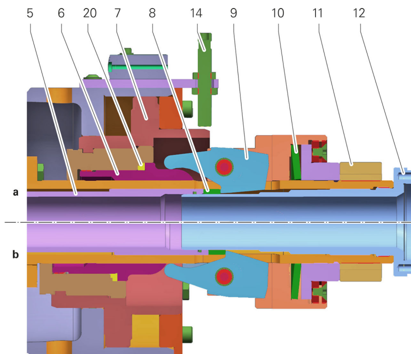
Knaggenspanneinrichtung_geöffnet/gespannt_TNL20
