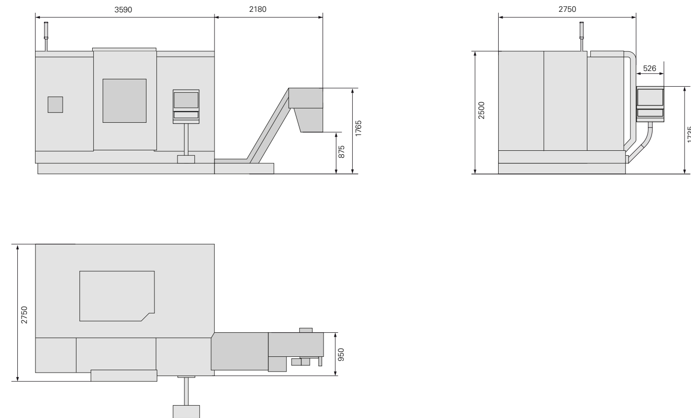
Plan d’implantation INDEX G200/G220 Convoyeur de copeaux sur le côté droit et manipulateur de pièces
