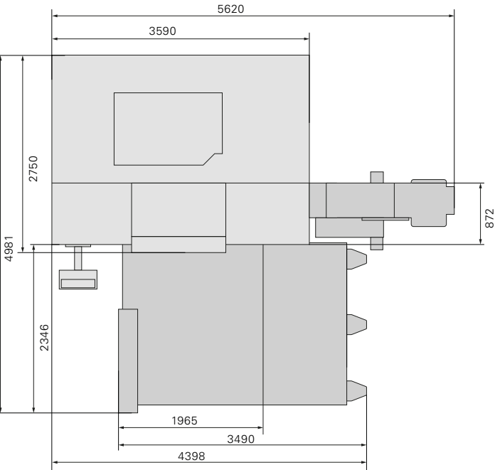
Plan d’implantation INDEX G200/G220 Convoyeur à copeaux sur le côté droit/ iXcenter L avec cellule de base et module à palettes
